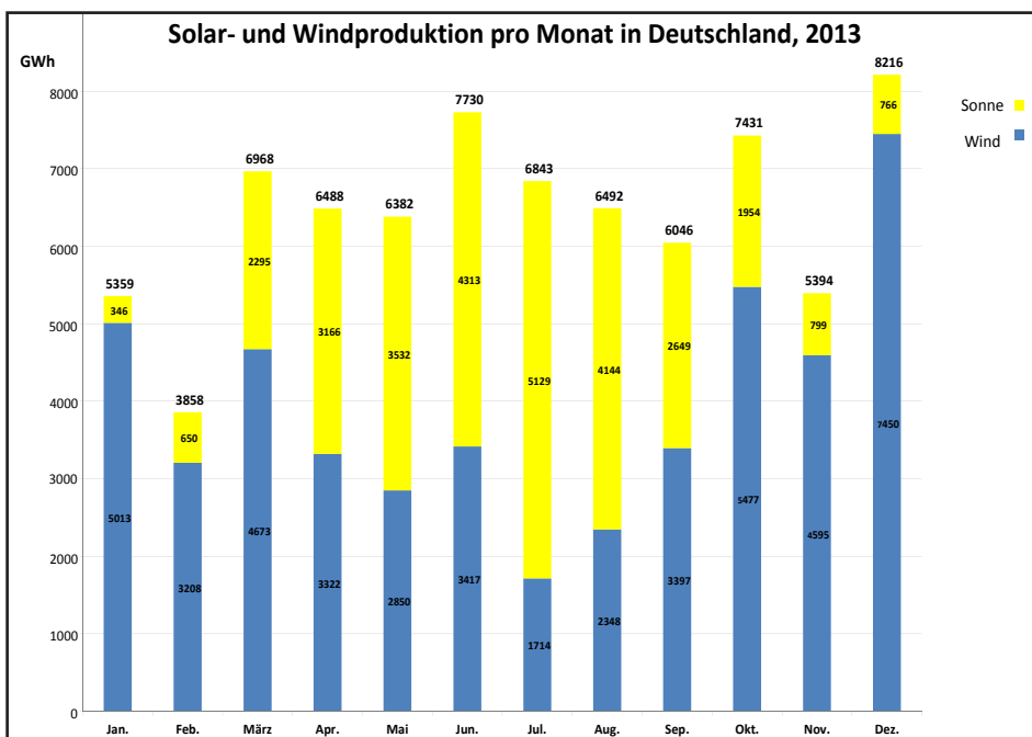
Abb. 5: Die Grafik zeigt, dass die stürmischen Winter in der Nordsee weitaus mehr Strom generieren als im Sommer. Wenn im Winter in der Schweiz das Wasser und die Sonne fehlen, kompensieren die Windanlagen in Deutschland den fehlenden Strom. (Quelle: European Energy Exchange. www.eex.com)
