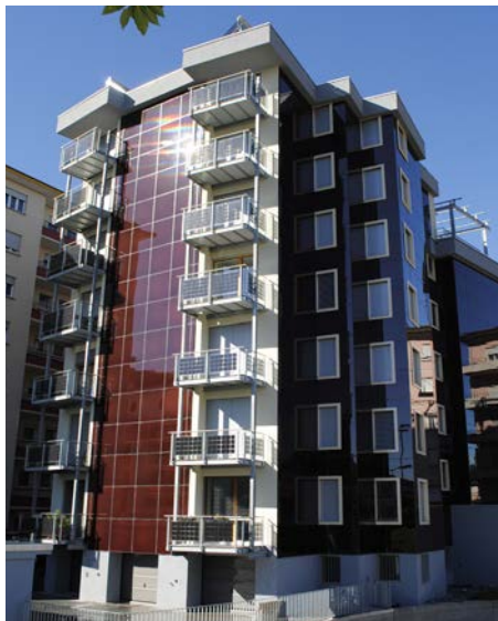
Abb. 3: Dank Minergie-P-Sanierung reduzierte dieses Mehrfamilienhaus in Chiasso/TI von 1965 seine Energieverluste um 88% und produziert mit Dach- und Fassadensolaranlage sogar 14% mehr Strom, als es selbst braucht. (Foto: Solar Agentur Schweiz)
